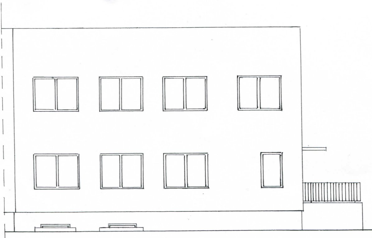
ELEWACJA PÓŁNOCNA c.d.
